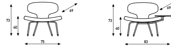
F 230 Libel
